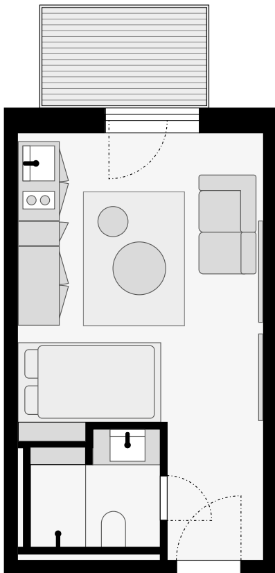
Beispiel-Grundriss
